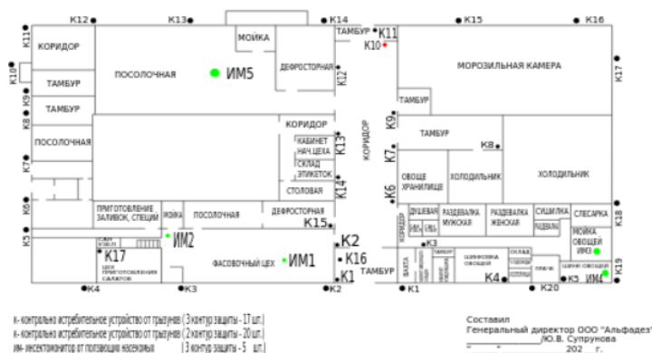
Схема расположения средств ПЕСТ контроля на предприятии ЗДАНИЕ : "РЫБНЫЙ ЦЕХ, 1 ЭТАЖ"
