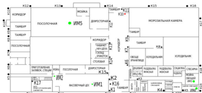
Схема расположения средств ПЕСТ контроля на предприятии ЗДАНИЕ : "РЫБНЫЙ ЦЕХ, 1 ЭТАЖ"
