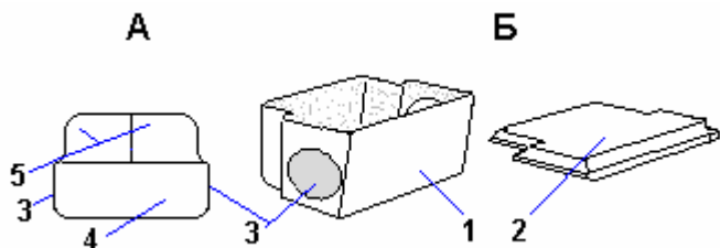
Рисунок. Емкость для работы с родентицидами. А – вид сверху внутри; Б – внешний вид.
